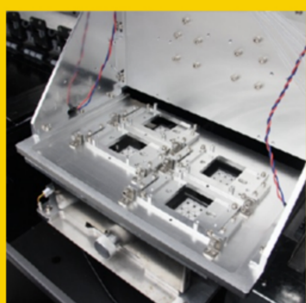
Carro del cabezal de impresión y sistema de calibración fabricados en aluminio para un ajuste físico preciso del cabezal de impresión y una configuración duradera.
